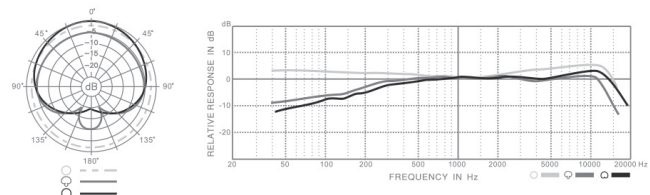
E309D PRO 频率响应图
