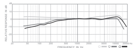
E309D PRO 頻率響應圖
